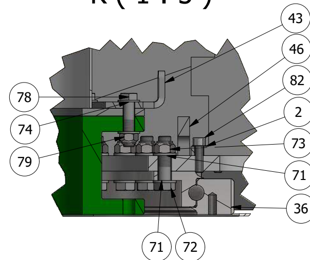
K ( 1 : 5 )
