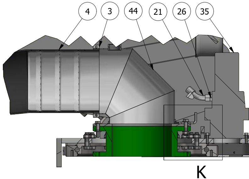
J ( 1 : 10 )
