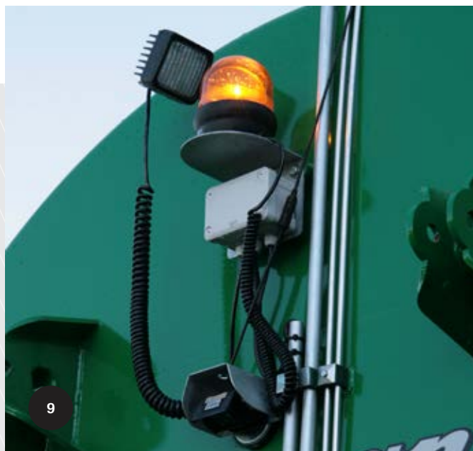
Rotorblinks-advarsel hjælper til med at undgå overfyldning af gyllevognen.
